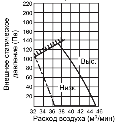
Производительность вентилятора <70Па>
