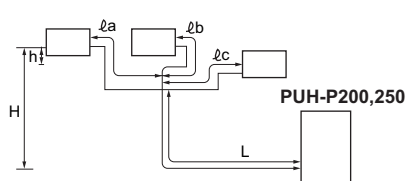
(3) Система «1 : 3»
