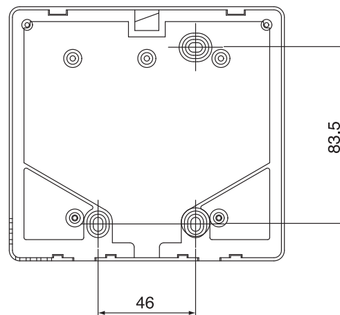
Вид сзади
