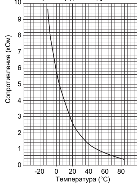
Термистор датчика дренажа
