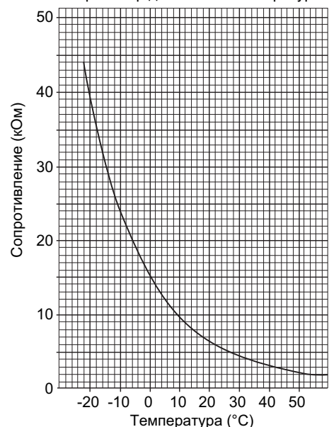
Термистор для низких температур
