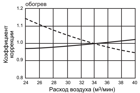
Производительность вентилятора <70Па>
