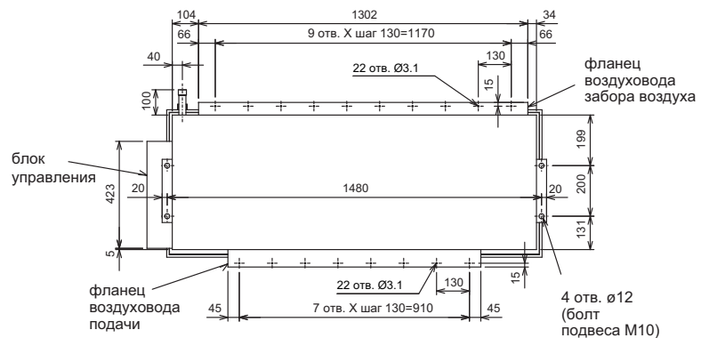
Вид сверху
