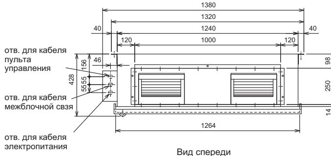
Вид спереди
