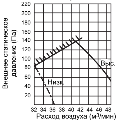
Производительность вентилятора <130Па>
