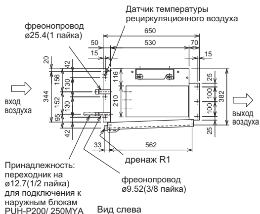
Вид слева
