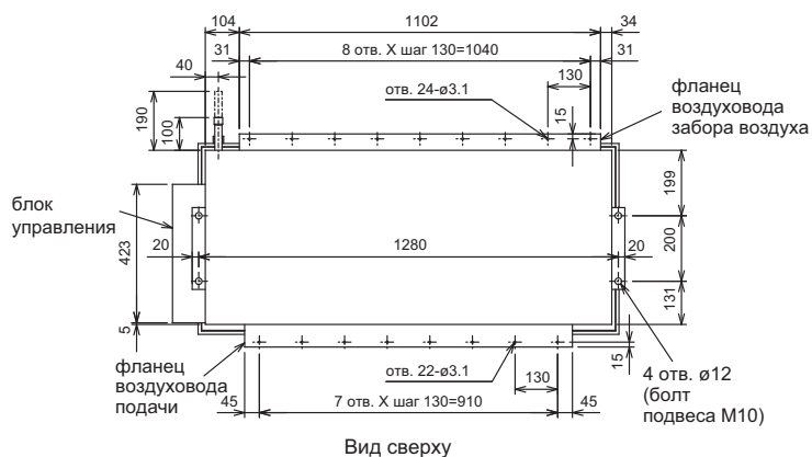
Вид сверху
